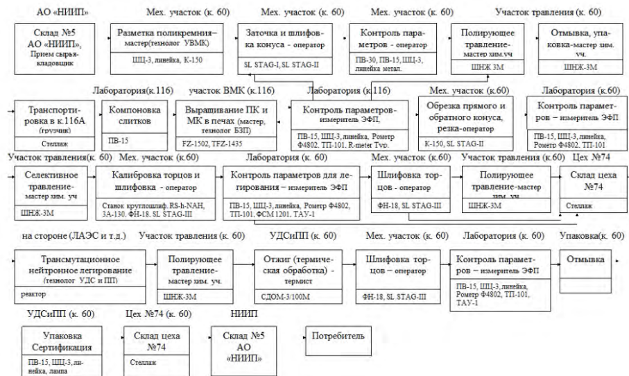
Схема 1 Технологическая схема производства монокристаллического кремния методом бестигельной зонной плавки
