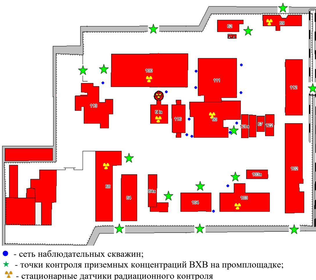
Рисунок 2. Схема санитарно-защитной зоны с указанием точек радиационного и химического контроля на промплощадке АО «НИИП»
